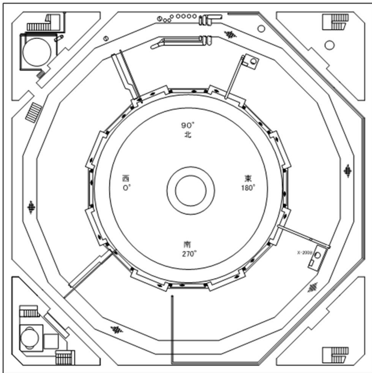
1号機 R/B 中地下階
