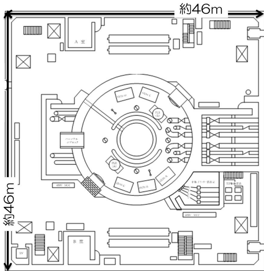
2号機 R/B 1階
