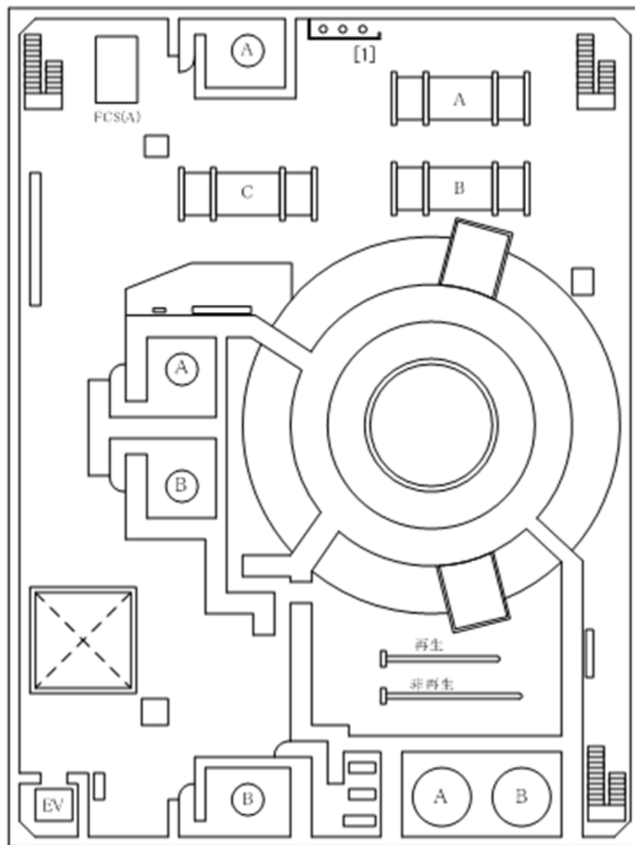
2号機 R/B 2階
