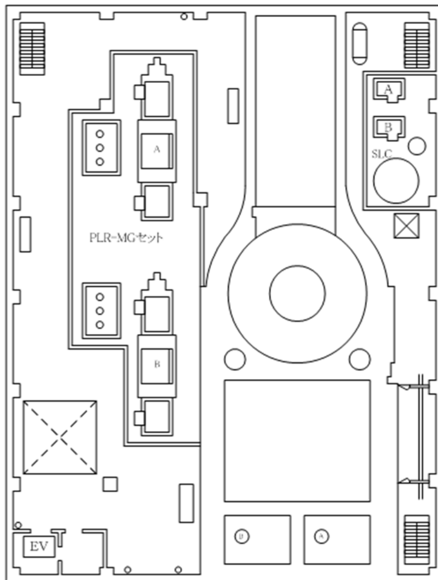
2号機 R/B 4階
