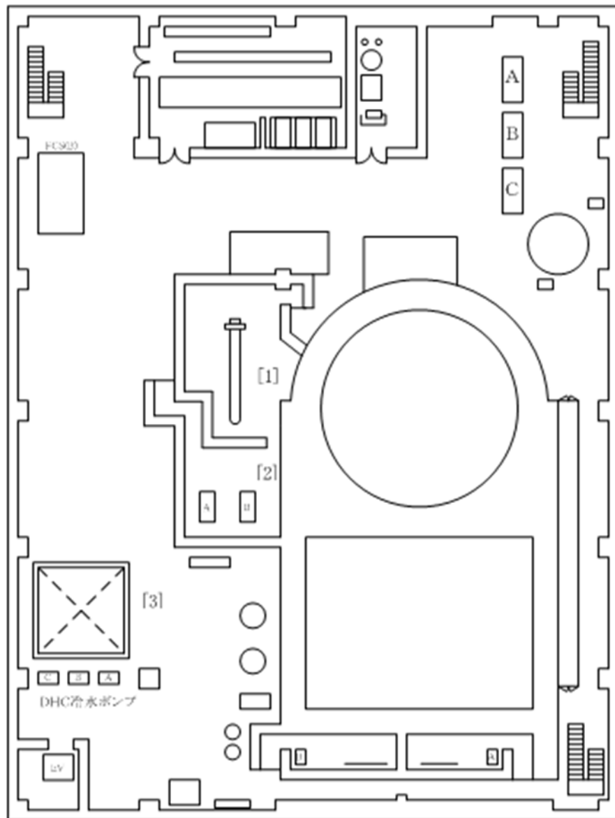
2号機 R/B 3階
