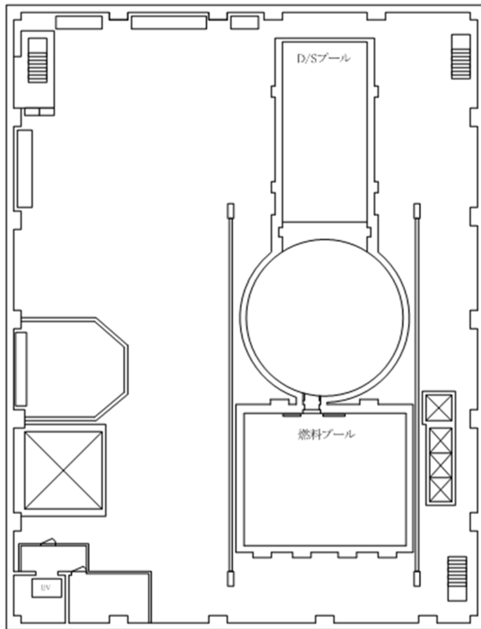
2号機 R/B 5階
