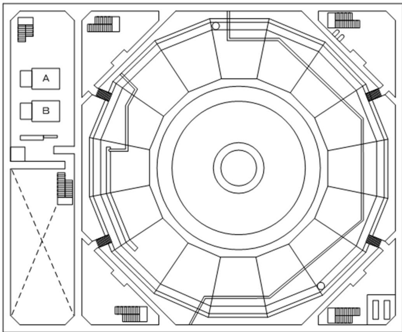
3号機 R/B 中地下階
