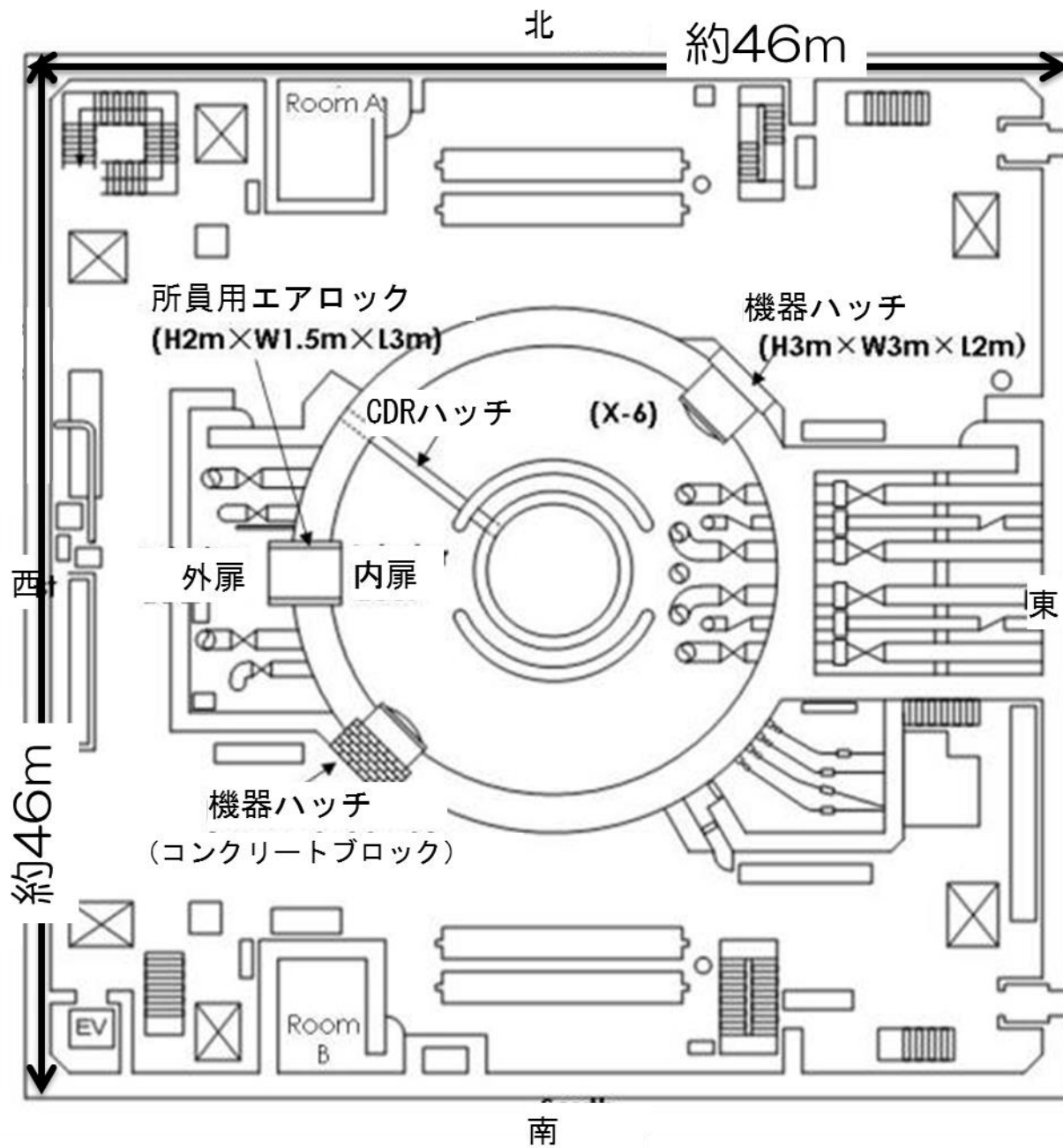
3号機 R/B 1階
