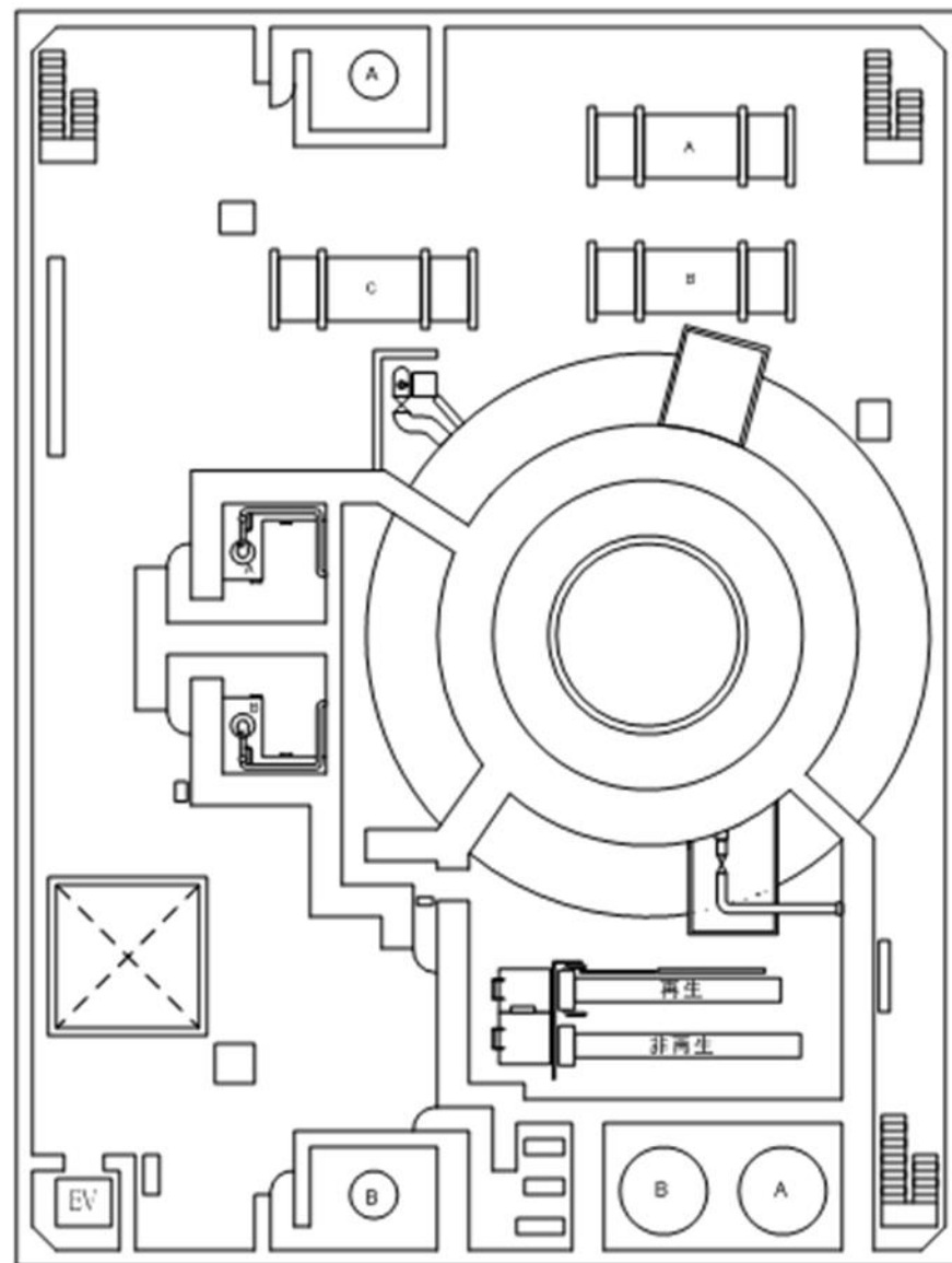
3号機 R/B 2階
