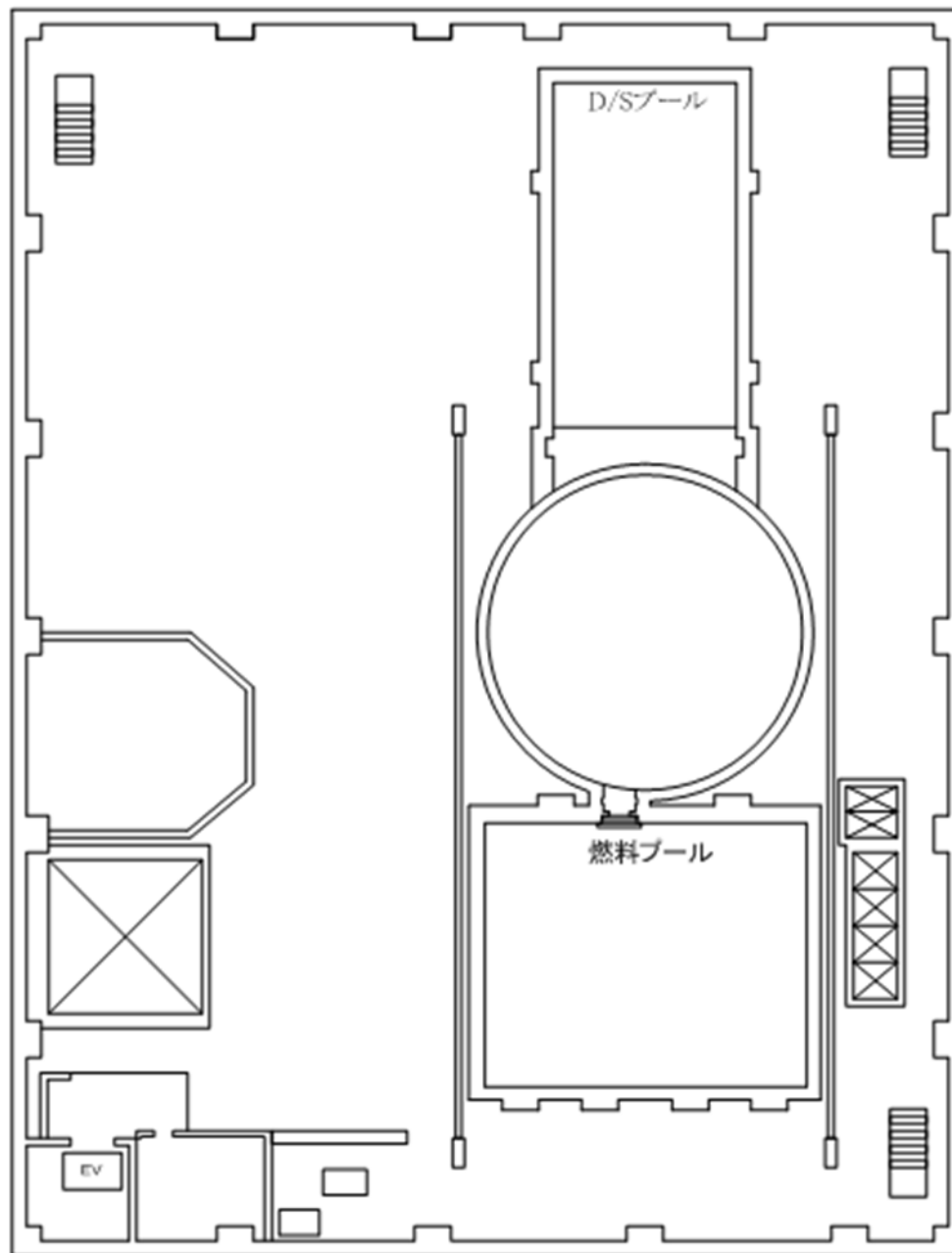
3号機 R/B 5階
