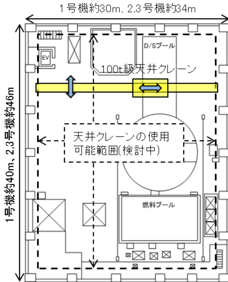
高さ方向の使用可能範囲 (オペフロ床～クレーンガータ下端は約8m)
