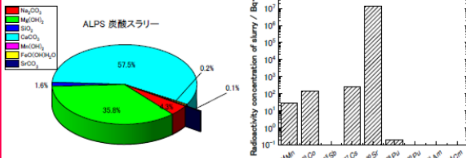
既設ALPSの炭酸沈殿物の分析結果 (JAEA)
