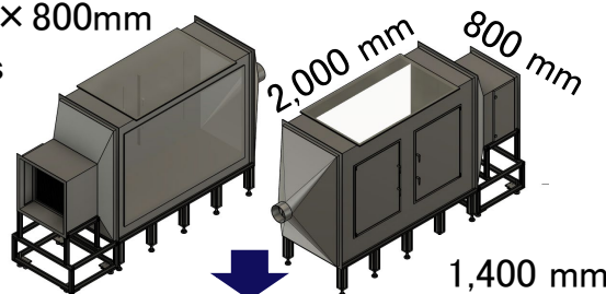
ケーシング3号機(詳細データ測定試験)
