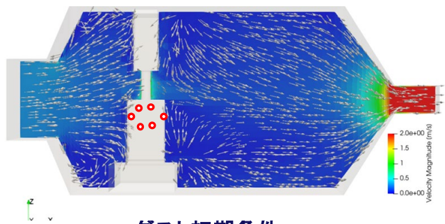
ダスト初期条件
