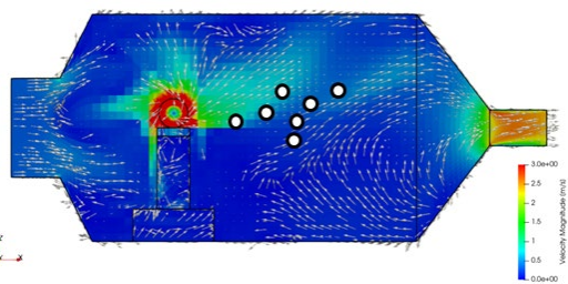
ダスト飛散挙動解析手法
