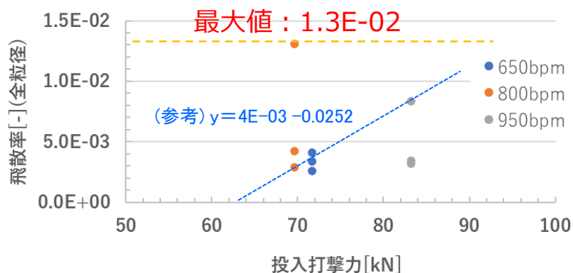
飛散率（ジルコン・平・20kg） <全粒径>
