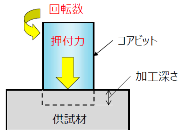
パラメータ補足説明図
