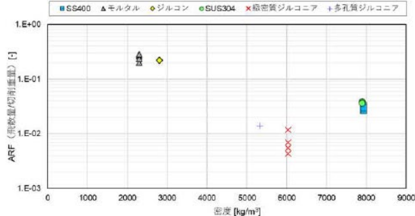
図 ARFと密度の関係
