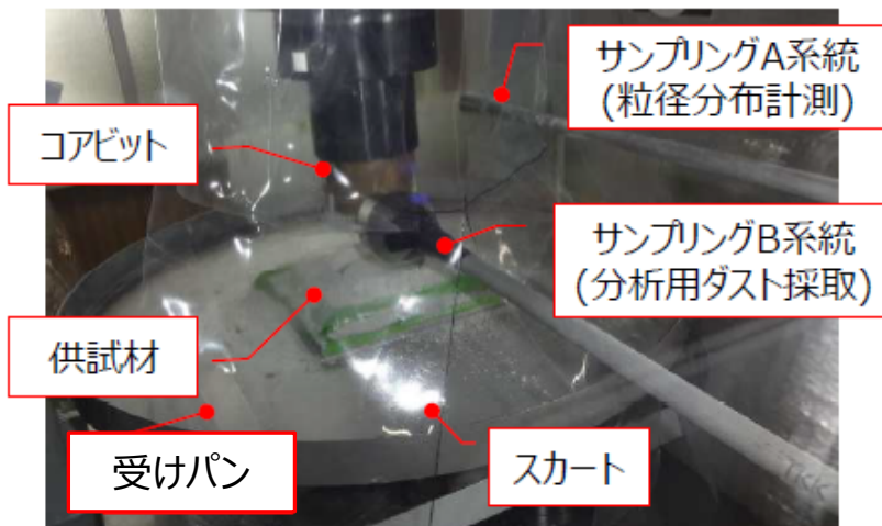
コアボーリング加工部外観
