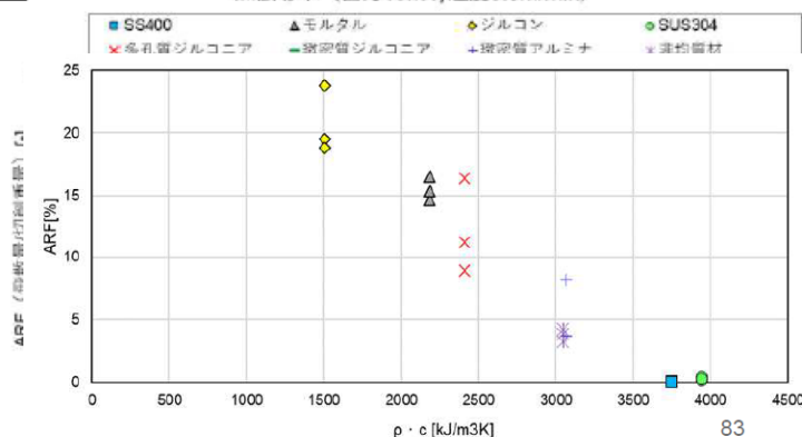
図 ARFと容積比熱の関係
