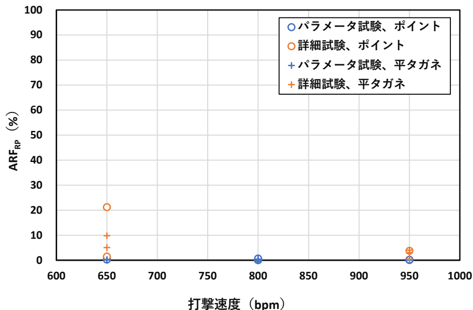
チゼルによるジルコン切削時の10μm以下粒子の飛散率 (ARF RP ) の打撃速度依存性
