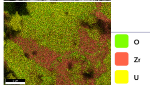
切削試験で飛散したダストの断面SEM-EDS
