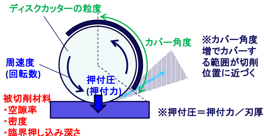
試験パラメータ 概略図
