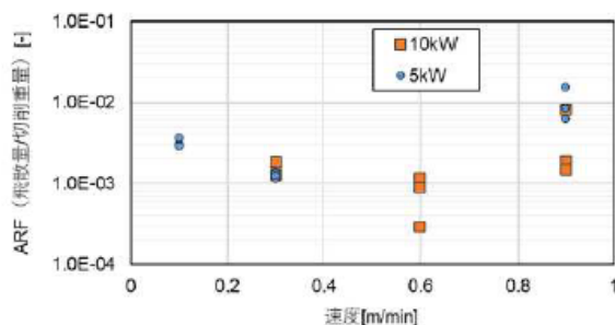
図 ARFと出力・速度の関係(SS400)
