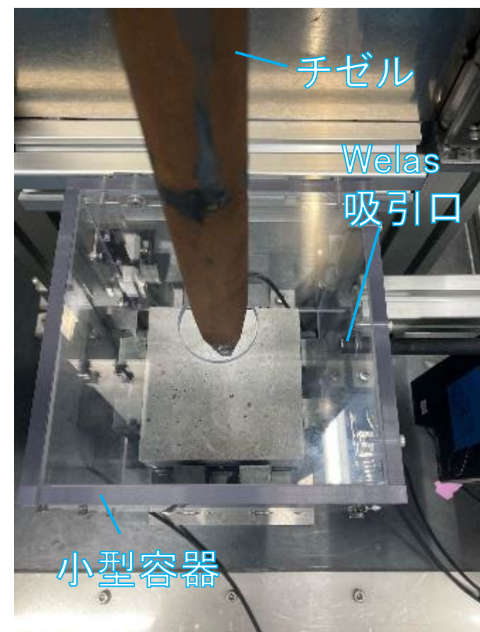
<試験体系(上から見た図)>
