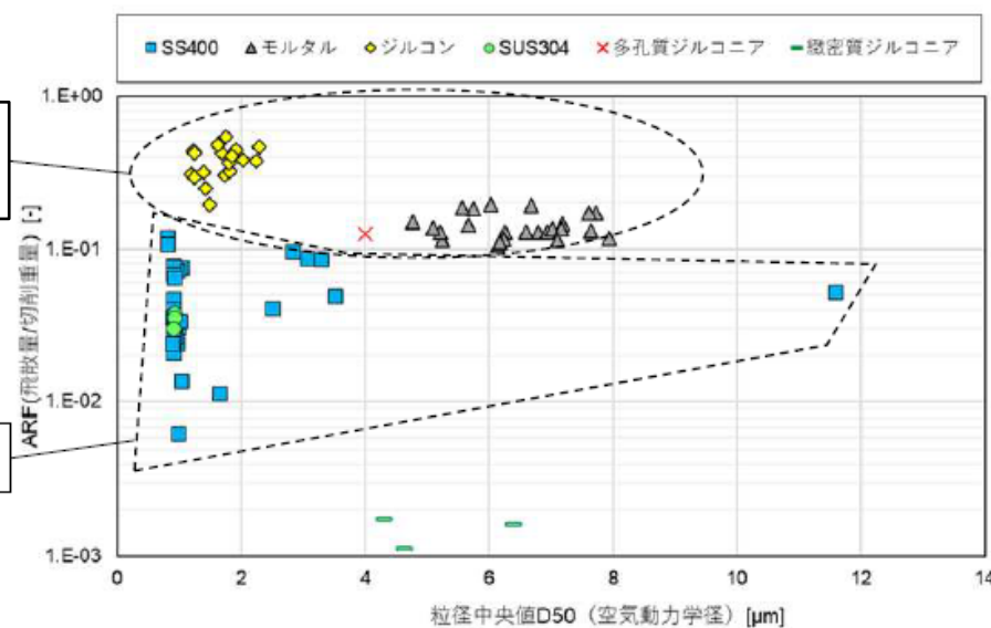
図 ARFとD50の関係（レーザー切断）
