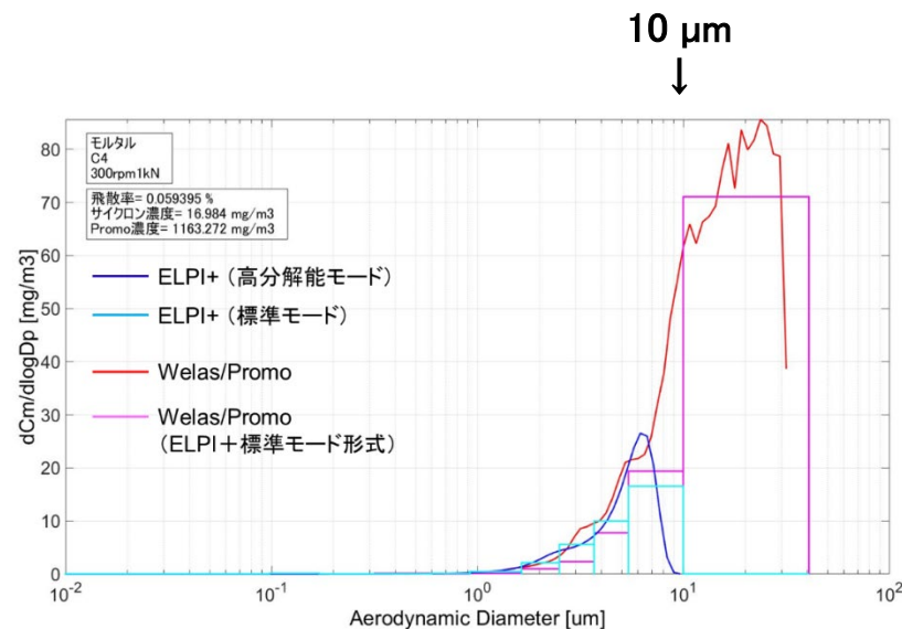
コアボーリングによるモルタル切削時の 飛散ダスト重量濃度の粒径分布 (空気動力学径換算)
