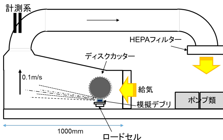
ダスト飛散率測定装置(NFD管理区域に設置)
