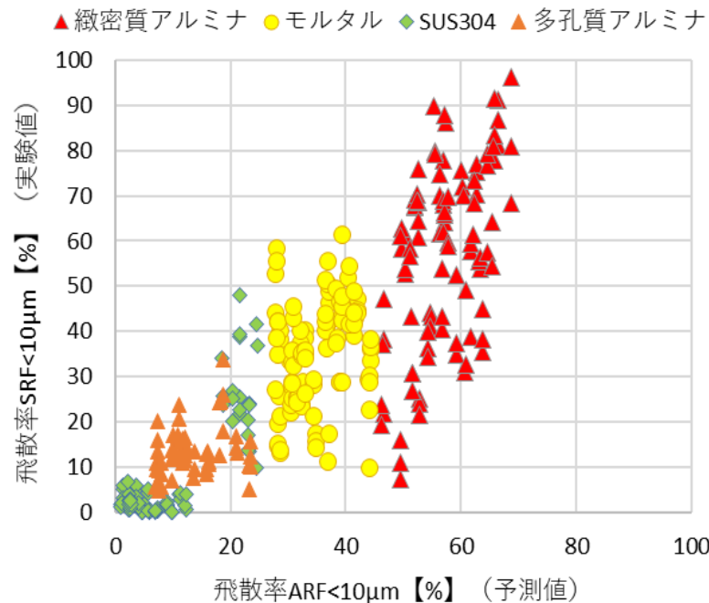
重回帰式による飛散率(10 \mu\text{m} 以下)の予測値と実験値
