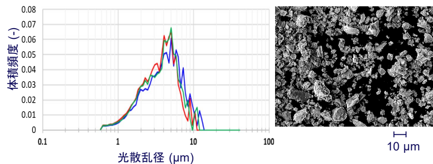
緻密質アルミナ
