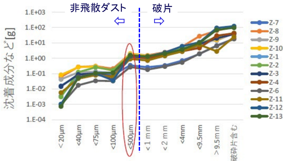
沈着粒子の分級結果(ジルコン、ポイントチゼル)
