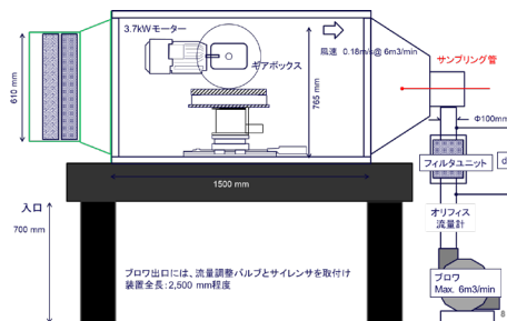
本事業のダスト飛散試験
