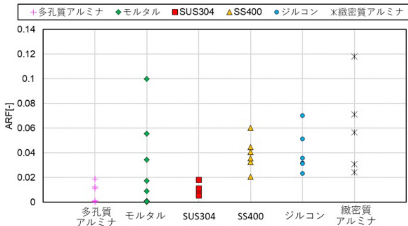
供試体毎のARF
