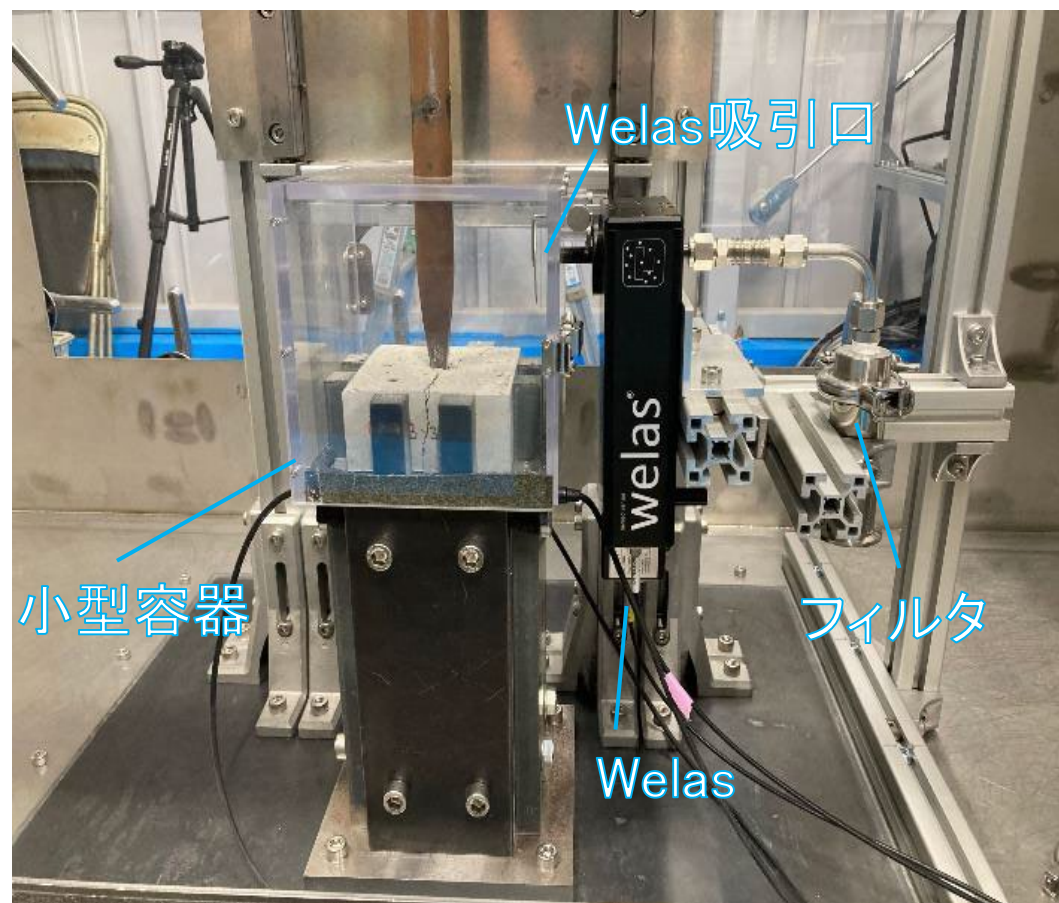
<試験体系(横から見た図)>
