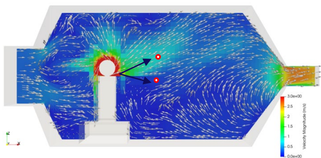
ダスト初期条件
