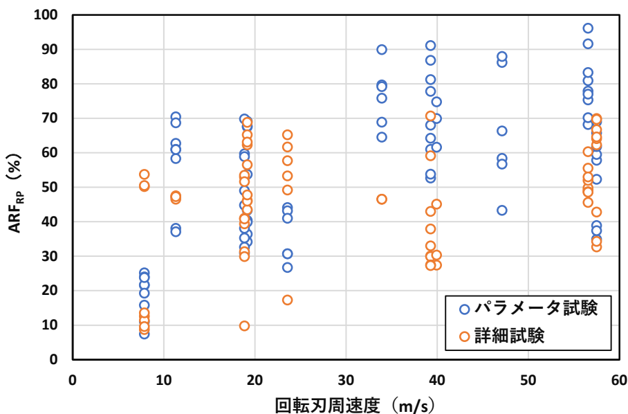
ディスクカッターによる緻密質アルミナ切削時の10μm以下粒子の飛散率 (ARF RP ) の周速度依存性
