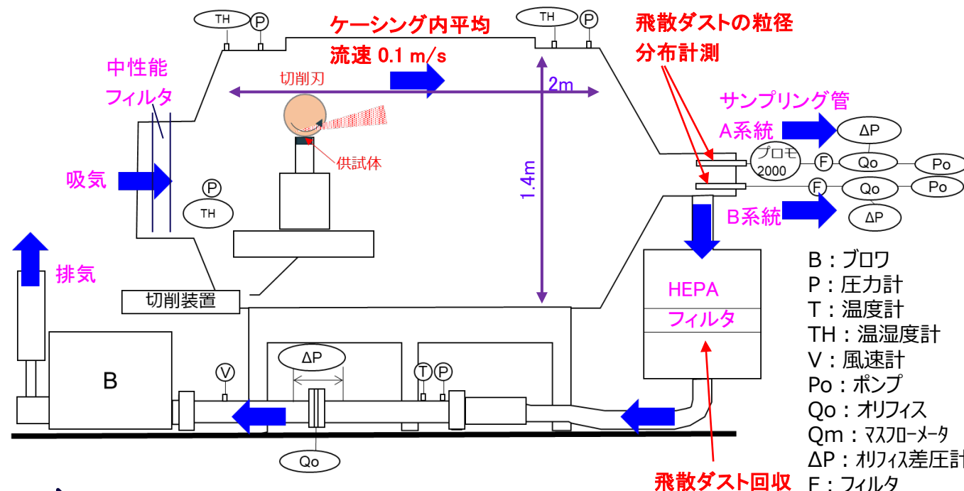
試験装置の概略図
