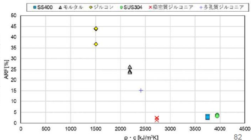
図 ARFと容積比熱の関係
