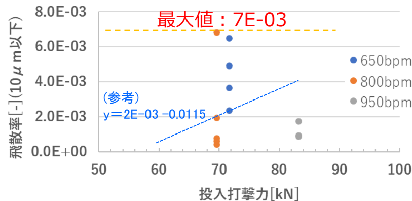
飛散率（ジルコン・ポイント・20kg） <10μm以下>
