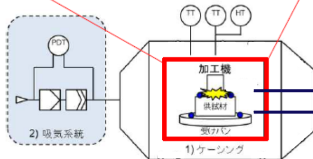
コアボーリング試験装置概略図
