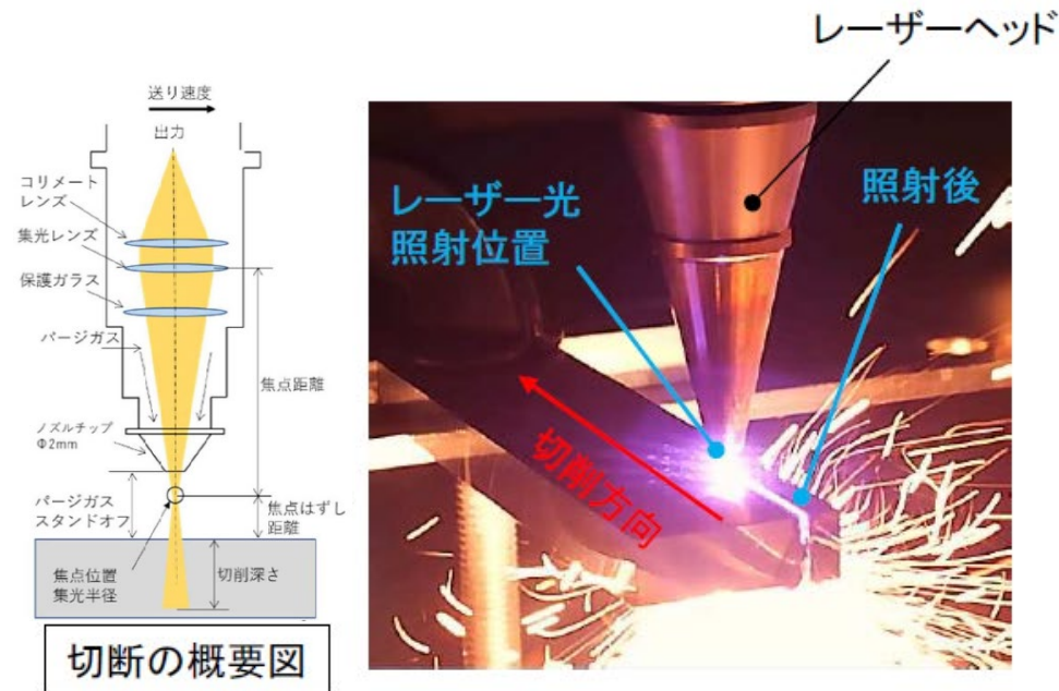
図 レーザー切断中の様子(SS400)
