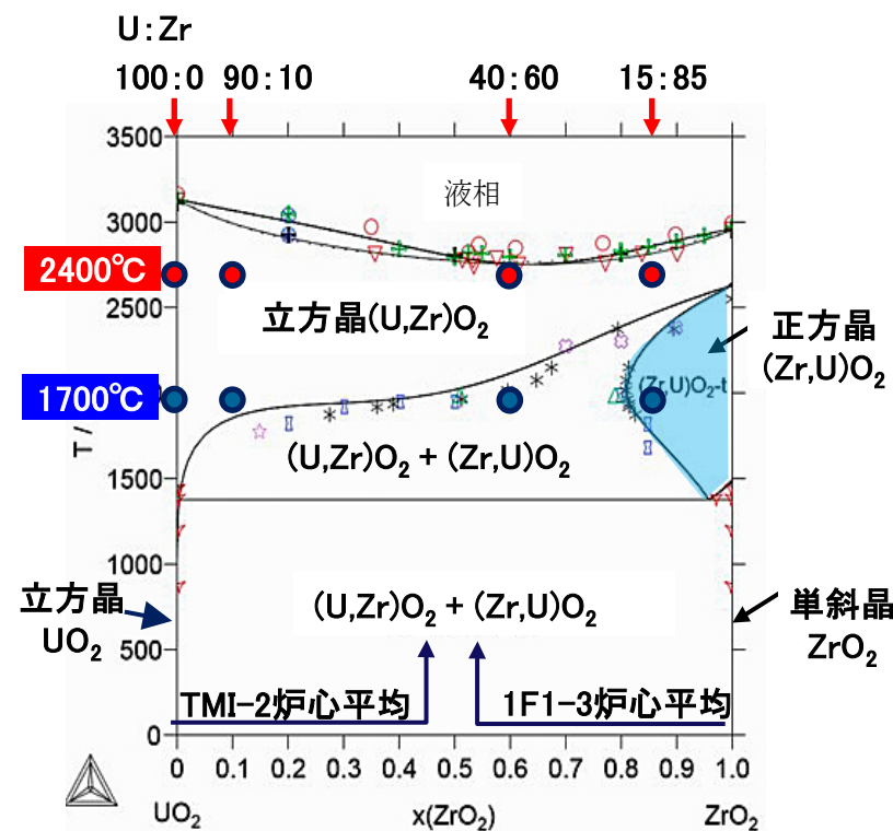
UO_2-ZrO_2 擬二元系状態図
