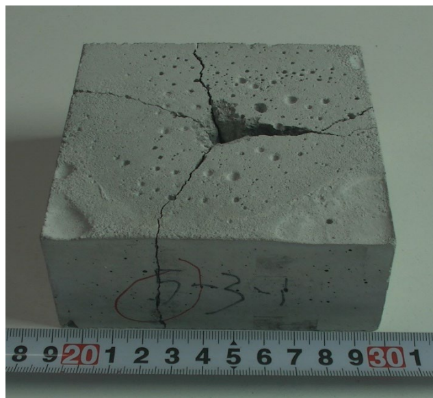
破碎後の供試体
