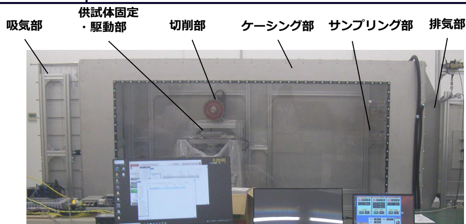
ダスト飛散率詳細データ測定装置
