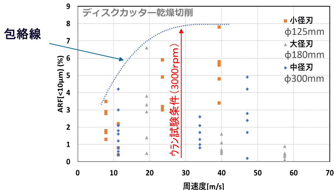
SUS304のディスクカッター切削による飛散率 ARF_{RP}
