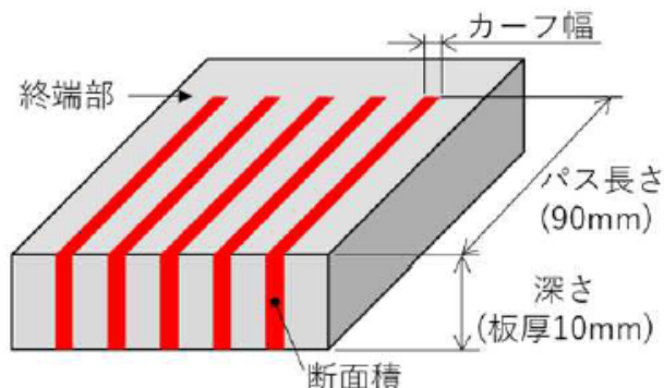
図 切断における深さとカーフ幅
