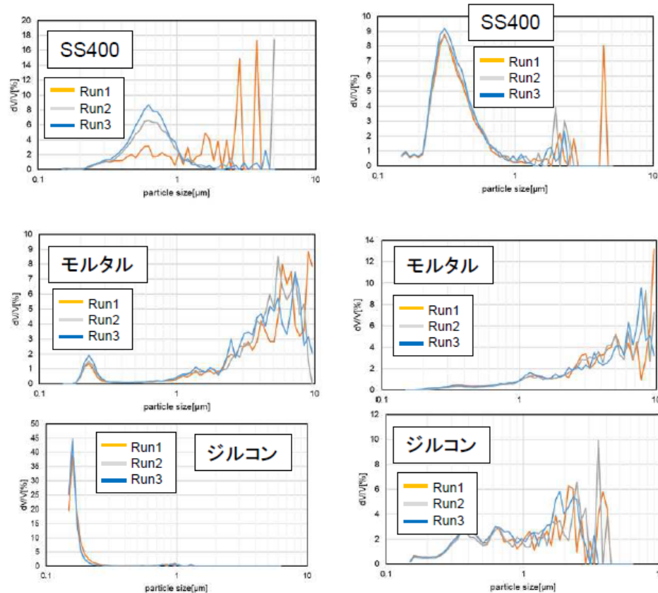
図 粒径分布の例(ガウジング)
