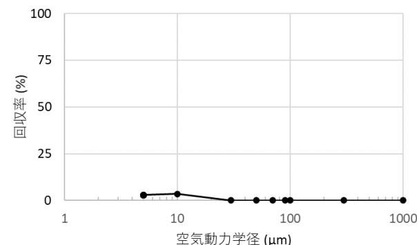
粒径ごとの回収率
