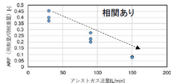
図 ARFとアシストガス流量の関係(モルタル)
