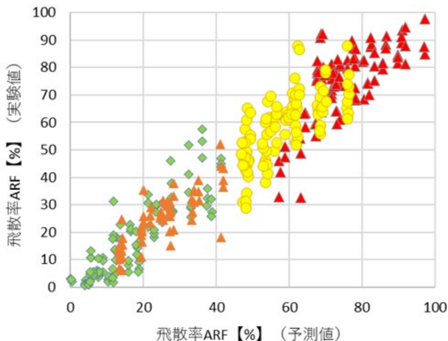
重回帰式による飛散率の予測値と実験値
