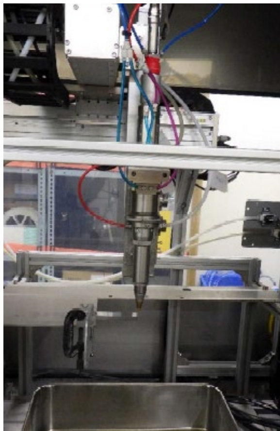
切削モードのレーザートーチ
